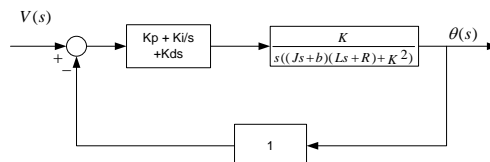
Gambar 13 Diagram blok loop tertutup pengontrol PID
