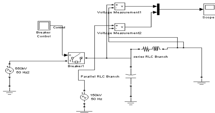
Gambar 9. Rangkaian simulasi tegangan implus transformator daya 150 kV
