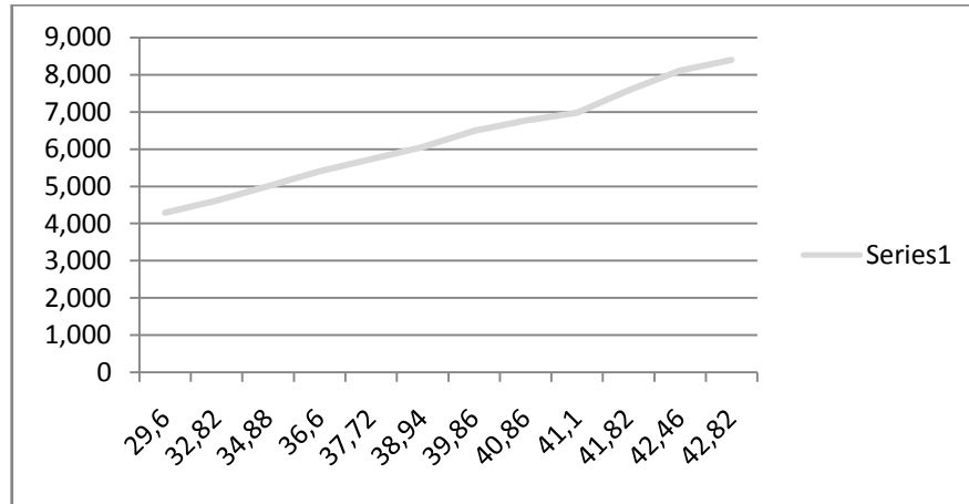
Gambar 1. Grafik hubungan daya keluaran dan temperatur panel sel surya
