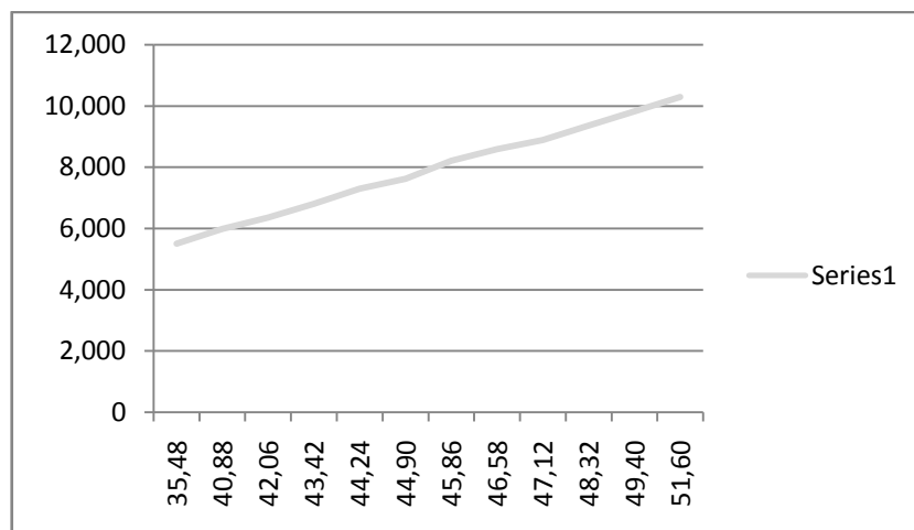
Gambar 2. Grafik hubungan temperatur dan daya keluaran setelah cahaya dilewatkan kumpulan lensa
