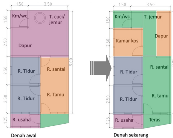
Gambar 3. Rumah hunian satu lantai dengan aksesibilitas sama (Sumber: Hasil survey dan analisa, 2011)
