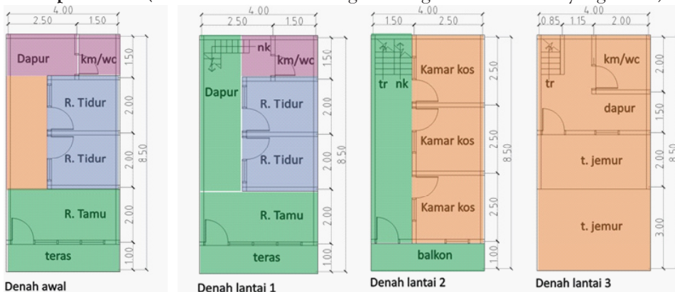
Gambar 5. Rumah hunian bertingkat dengan aksesibilitas yang sama (Sumber: Hasil survey dan analisa, 2011)
