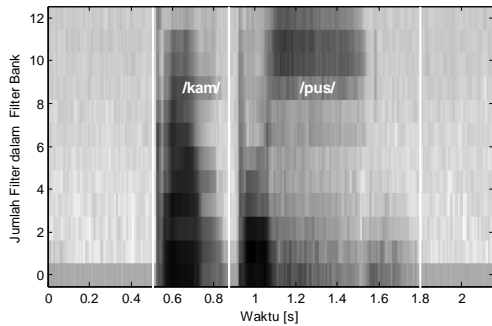
Gambar 16. Spektrum daya dimodifikasi dengan mel cepstral filter ( M=100 , N=256 ).
