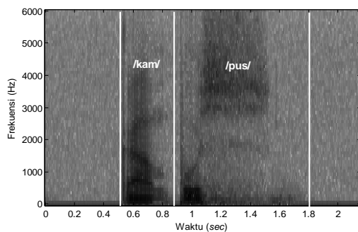
Gambar 12. Spektrogram sinyal wicara /kampus/, M = 50 dan N = 128 .
