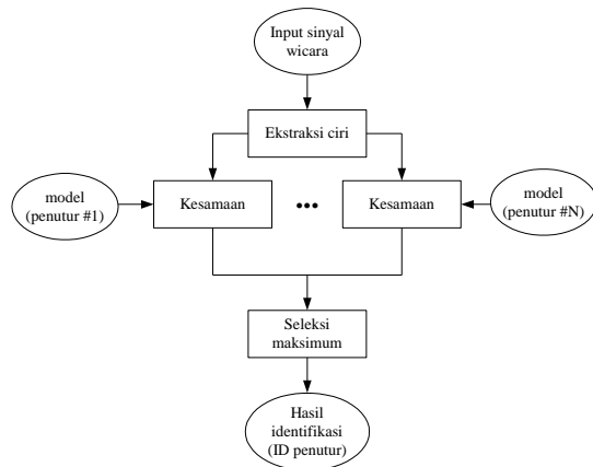
Gambar 1. Struktur dasar sistem pengenalan penutur
