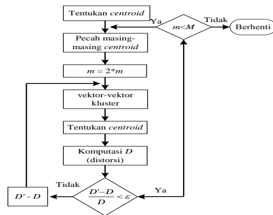
Gambar 6. Diagram alir algoritma LBG.
