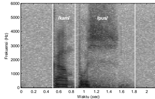
Gambar 14. Spektrogram sinyal wicara /kampus/, M = 200 dan N = 512 .
