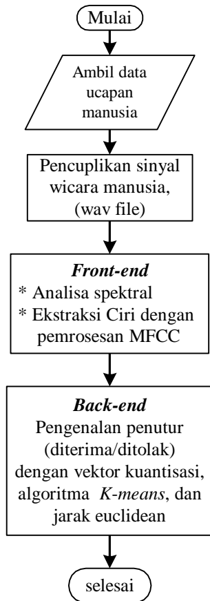
Gambar 8. Diagram alir sistem pengenalan penutur dengan metode mel-frequency .
