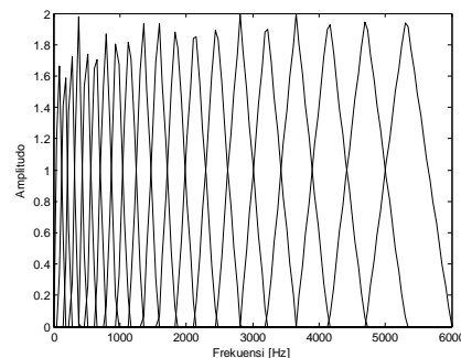
Gambar 15. Hasil filter bank dalam proses mel frekuensi.
