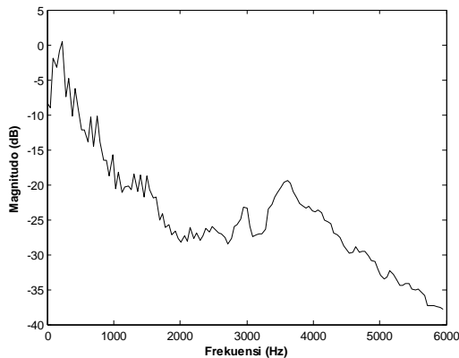
Gambar 11. Spektum sinyal dengan panjang window , N = 256 dan M = 100 pada kata /kampus/.
