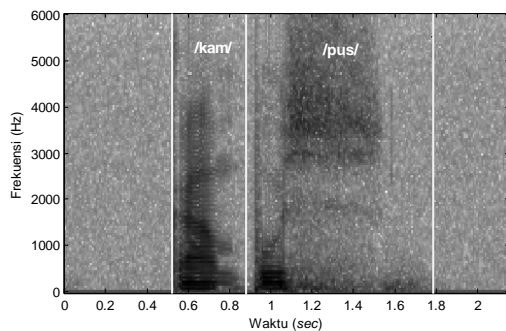
Gambar 13. Spektrogram sinyal wicara /kampus/, M = 100 dan N = 256 .
