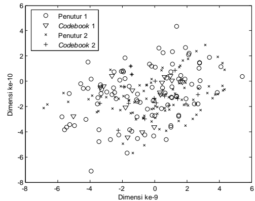
Gambar 18. Sebaran vektor-vektor akustik dari dua penutur dan codebook -nya, mfcc 12, filter bank 20, dan 16 centroid ( N=256 , M=100 ).
